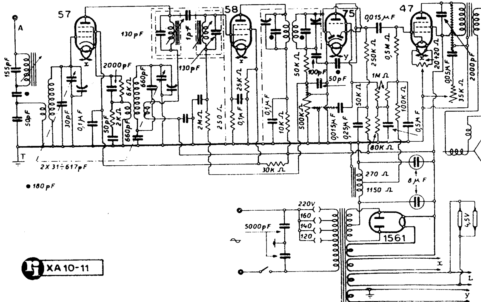
F.I.M.I. - MOD. PHONOLA « 790-1 »
